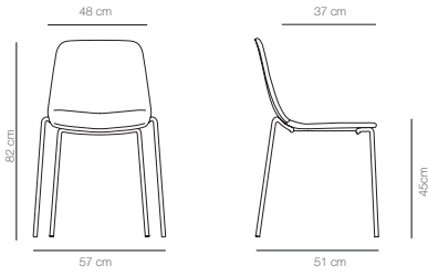
MAAL4P - Silla cuatro patas tapizado liso
