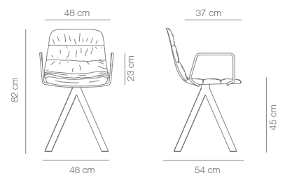
MAB - Brazos tapizado soft
