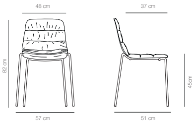
MAA4P - Silla cuatro patas tapizado soft
